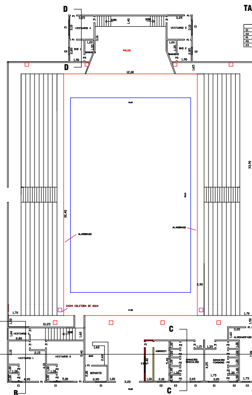
PLANTA BAIXA GINÁSIO DE ESPORTES (SITUAÇÃO ATUAL)
